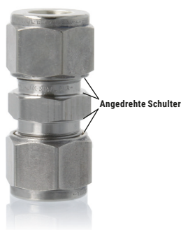
Metrische Verschraubung
