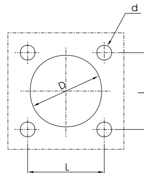
Gewindebohrungen im Gehäuse: M4, Tiefe 6 mm
